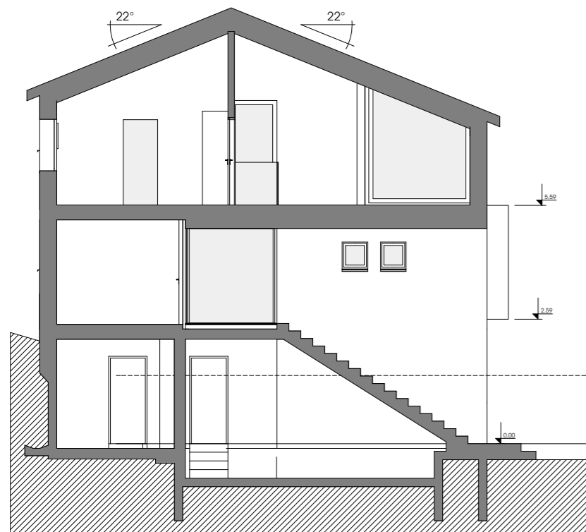
Schnitt Mst. 1:50
